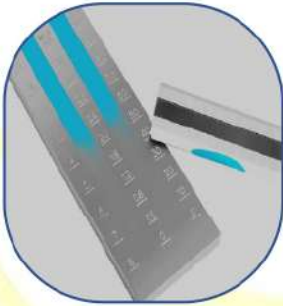
Hegman Gauge
